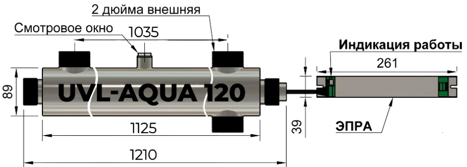
Рисунок 1. Габариты установки UVL-Aqua 120
