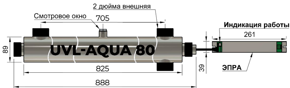
Рисунок 1. Габариты установки UVL-Aqua 80
