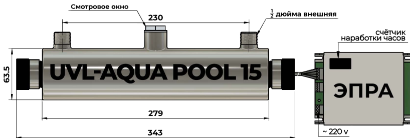
Рисунок 1. Габариты установки UVL-AQUA POOL 15
