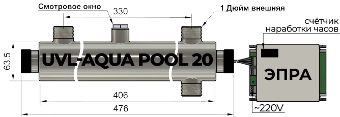
Рисунок 1. Габариты установки UVL-AQUA POOL 20
