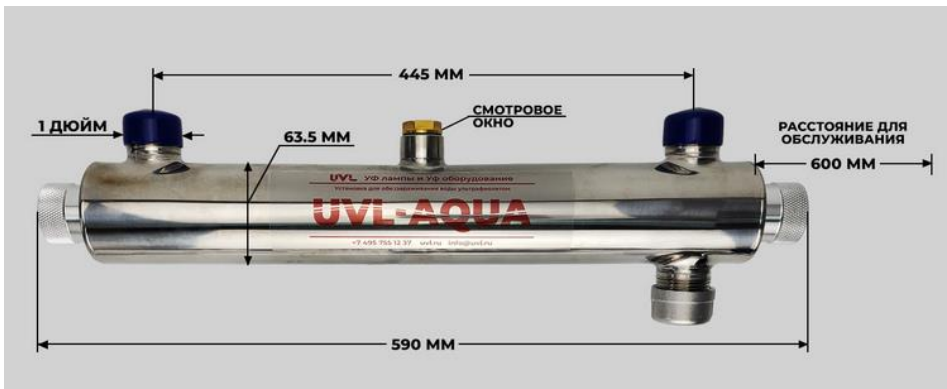
Рисунок 1. Габариты установки UVL-Aqua 28
