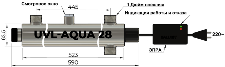
Рисунок 1. Габариты установки UVL-AQUA POOL 28
