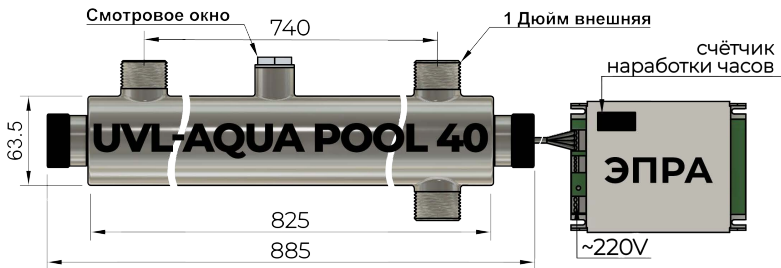
Рисунок 1. Габариты установки UVL-AQUA POOL 40
