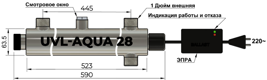
Рисунок 1. Габариты установки UVL-Aqua Hot 28
